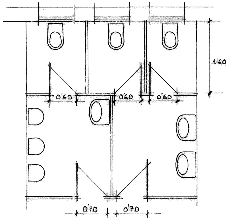
EN PROJECTE
